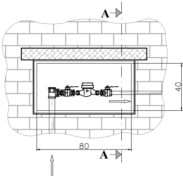
TLOCRT
