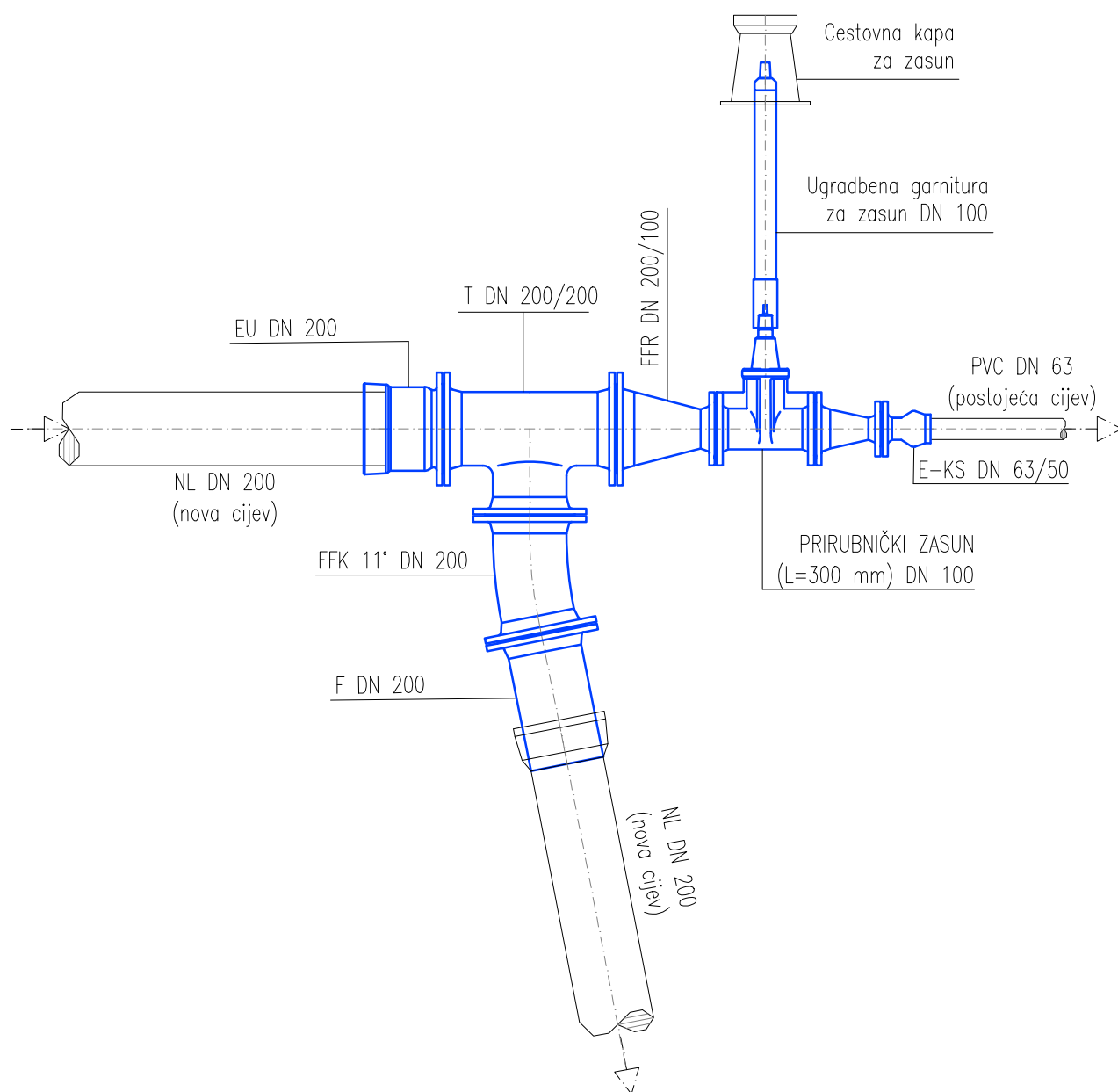
HEMA ČVORA 20 M 1:20
