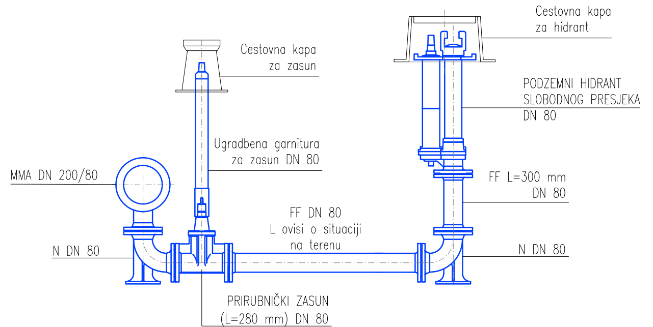
PRESJEK A-A
