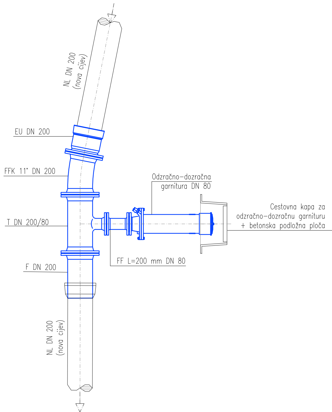
ŠEMA ČVORA 28 M 1:20
