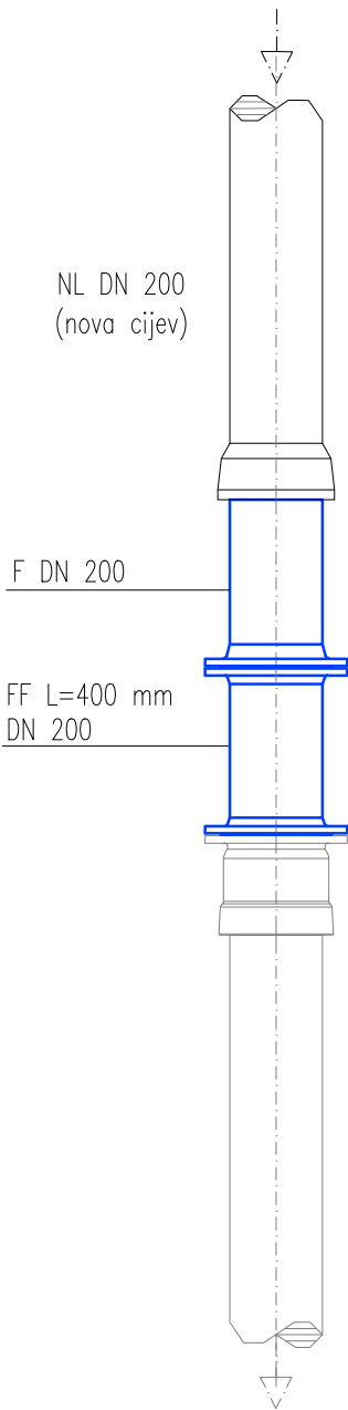
SHEMA ČVORA 35 M 1:20
